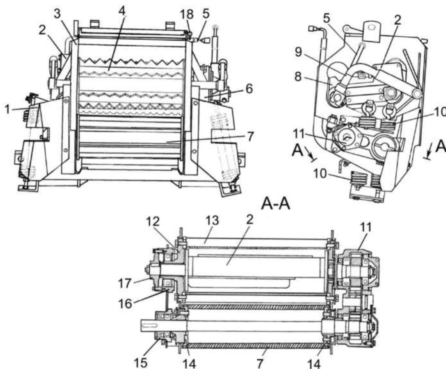
Рисунок 1.3 – Питающий аппарат
