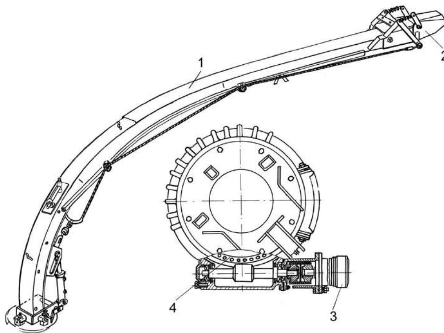
Рисунок 1.10 - Силосопровод
