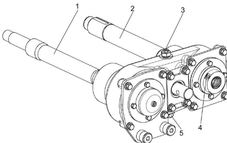
Рисунок 1.4 – Редуктор нижних валцов
